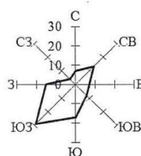
Повторяемость направления ветра, %. Год.
